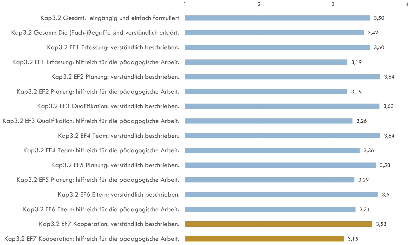
Kapitel 3.2 - Mittelwerte
